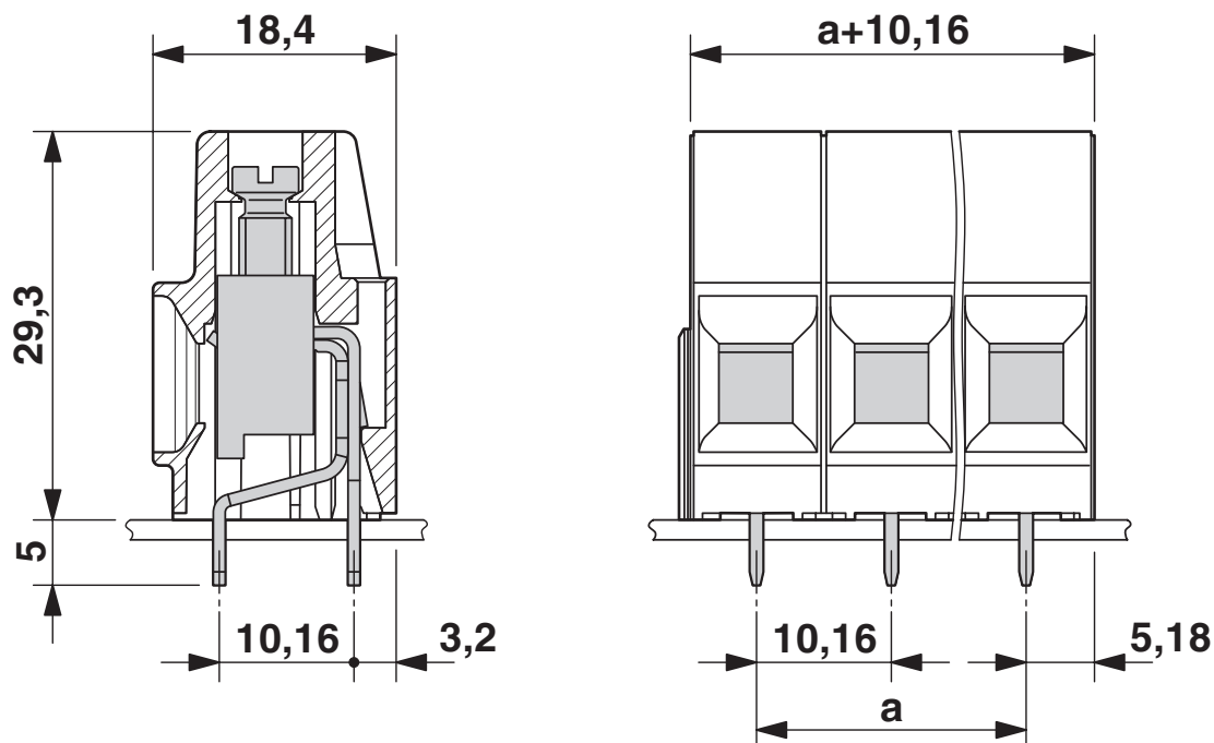
Måttskiss
