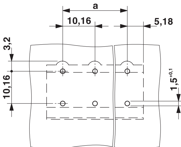
Borrplan/lödöns geometri
