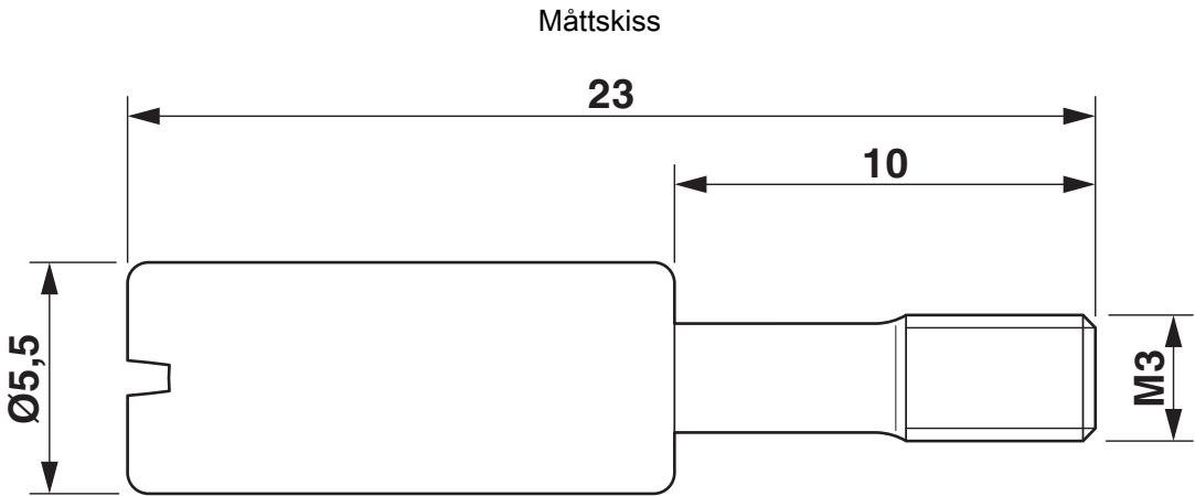
Schematisk ritning
