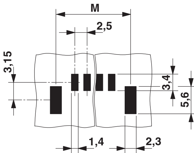
Borrplan/löddöns geometri
