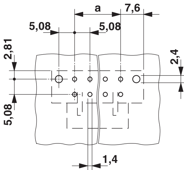
Borrplan/lödöns geometri
