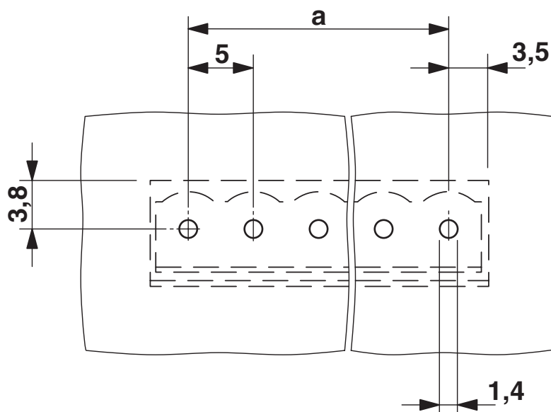
Borrplan/lödöns geometri
