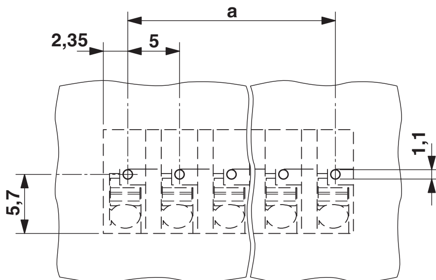
Borrplan/lödöns geometri
