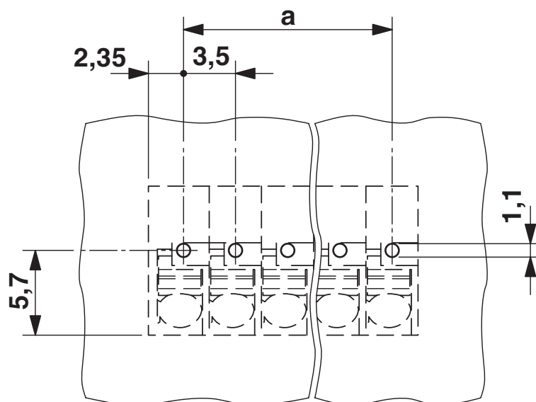
Borrplan/lödöns geometri
