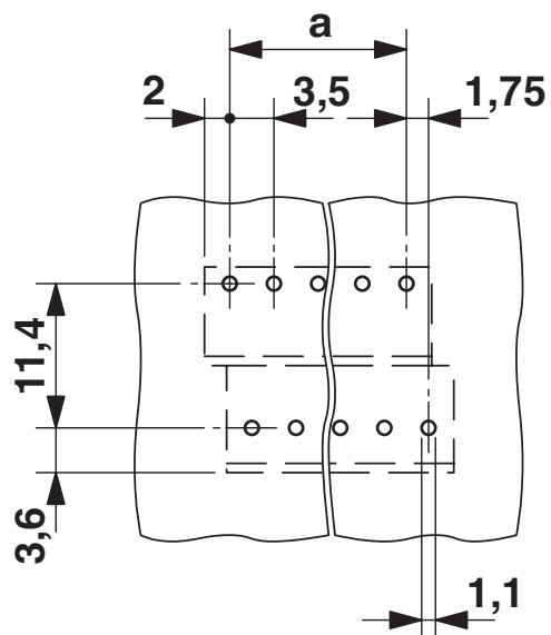
Borrplan/lödöns geometri
