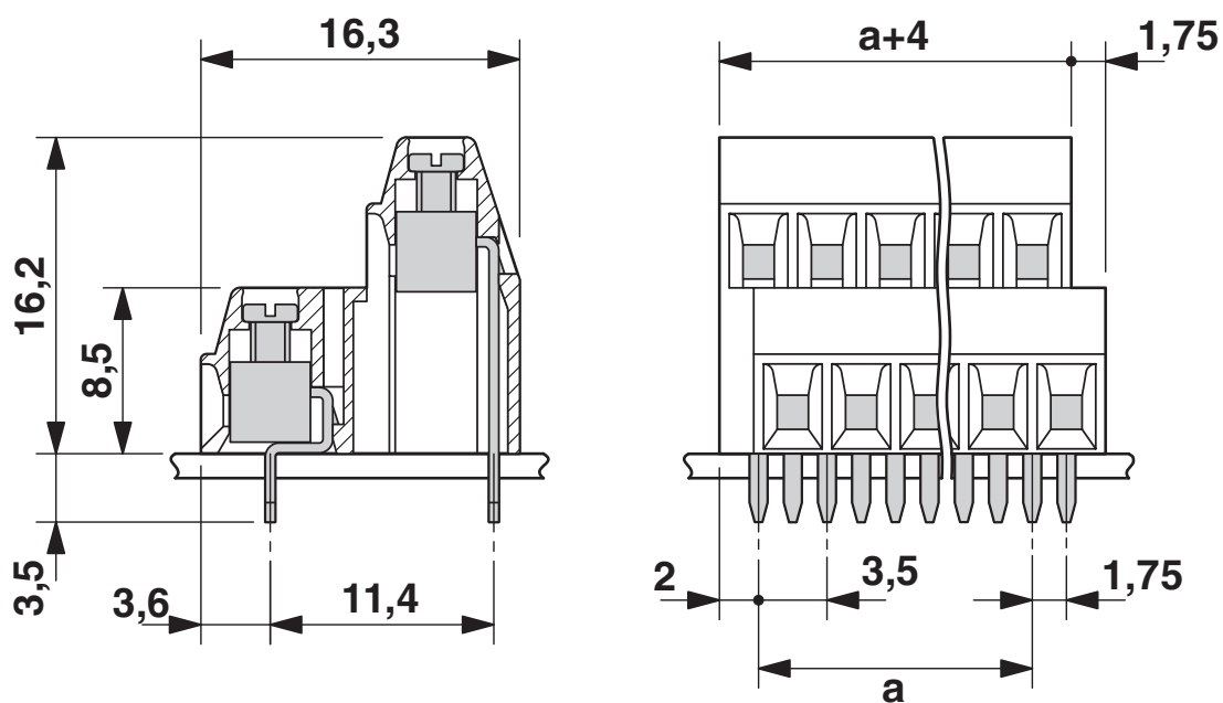
Måttskiss
