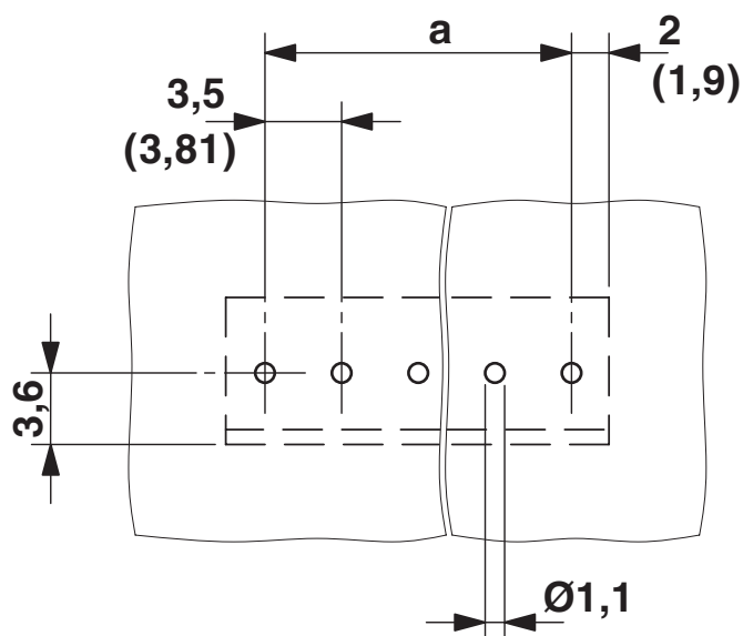
Borrplan/lödöns geometri
