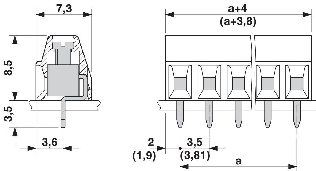
Måttskiss
