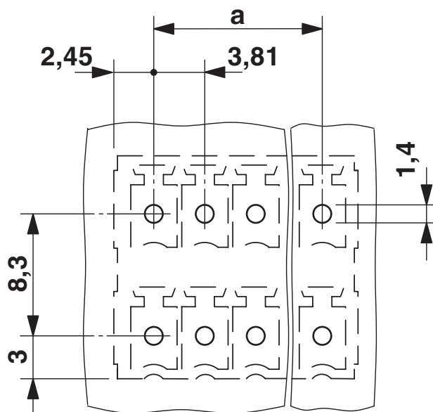
Borrplan/lödöns geometri
