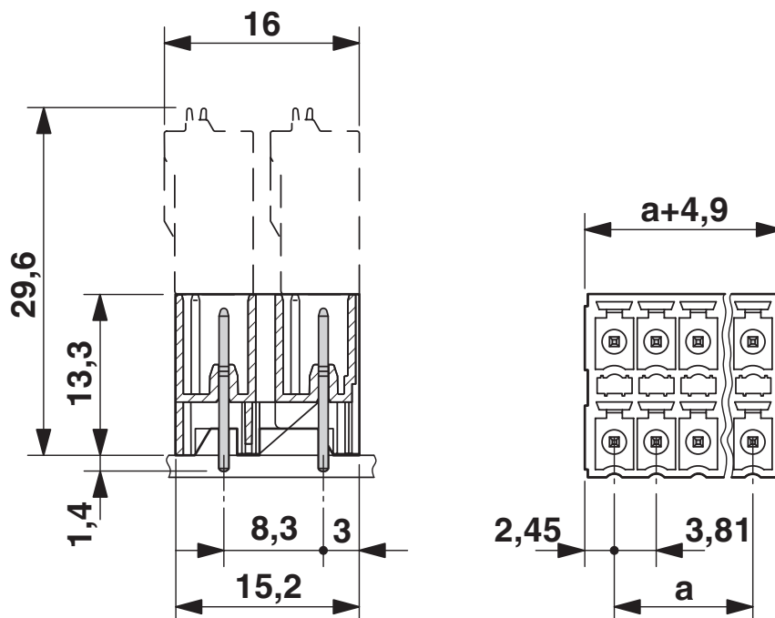
Måttskiss
