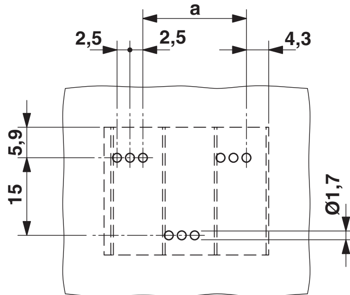
Borrplan/lödöns geometri
