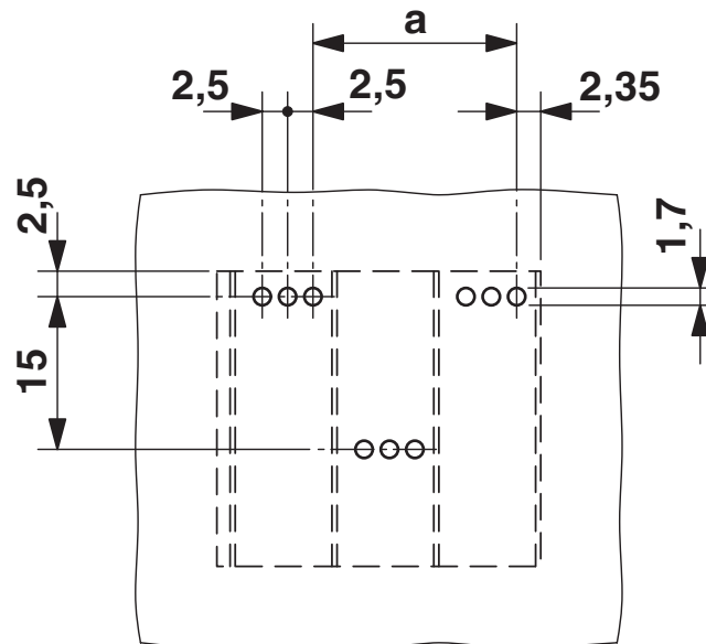
Borrplan/lödöns geometri
