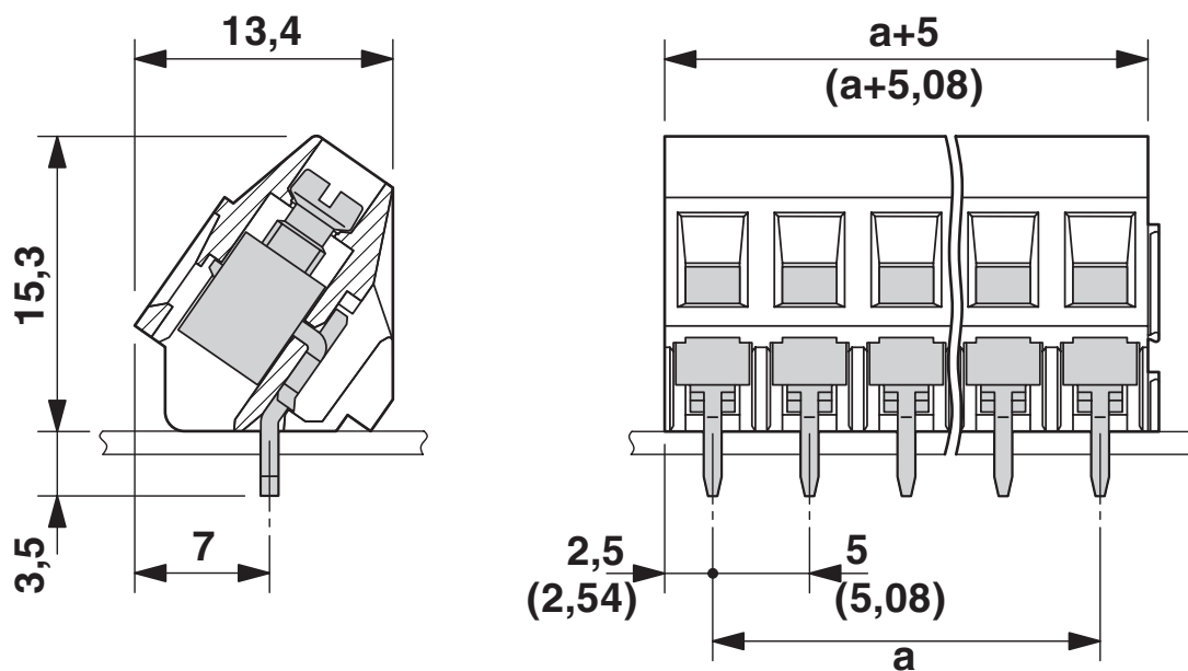
Måttskiss
