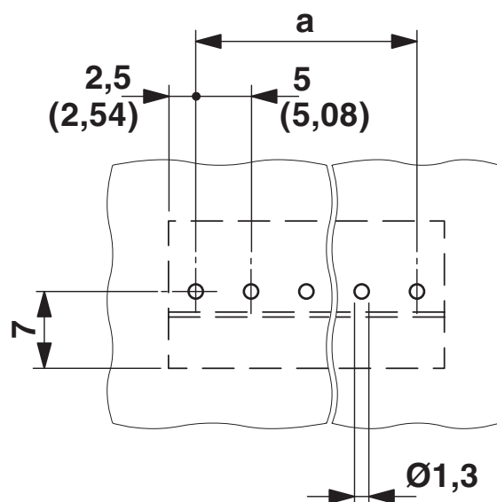
Borrplan/lödöns geometri
