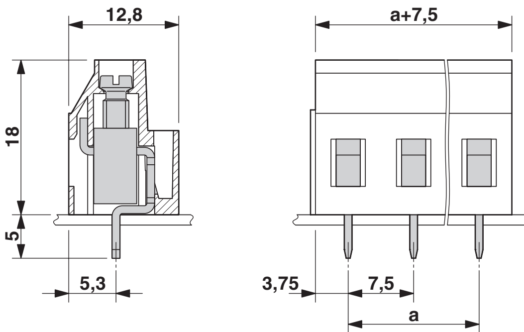
Måttskiss
