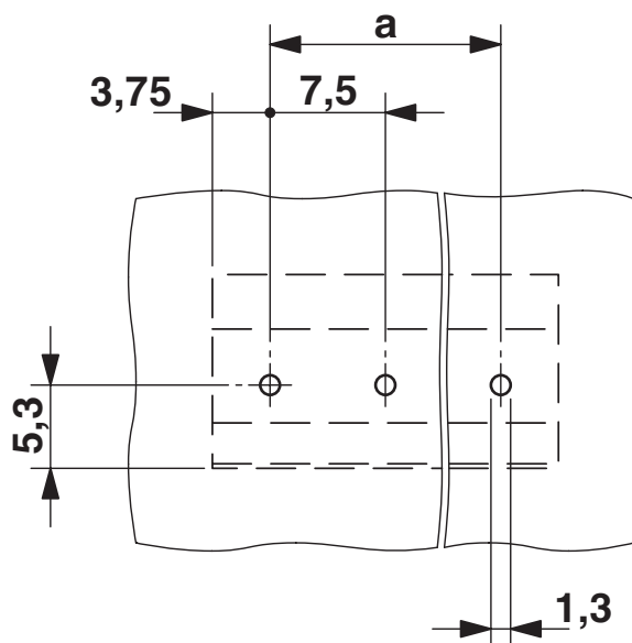
Borrplan/lödöns geometri
