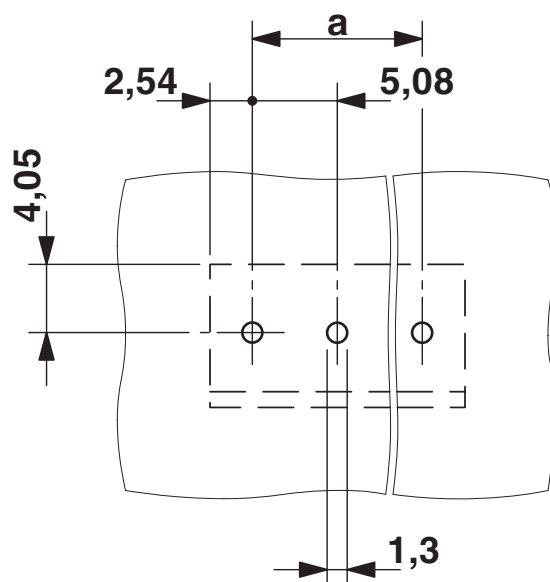
Borrplan/lödöns geometri
