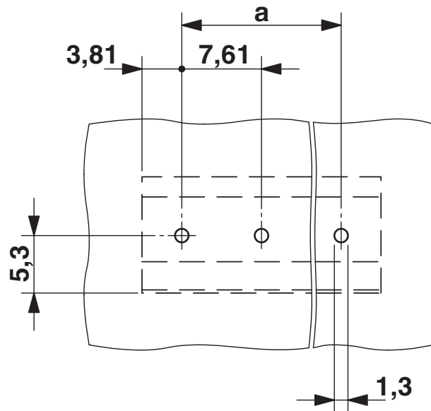
Borrplan/lödöns geometri
