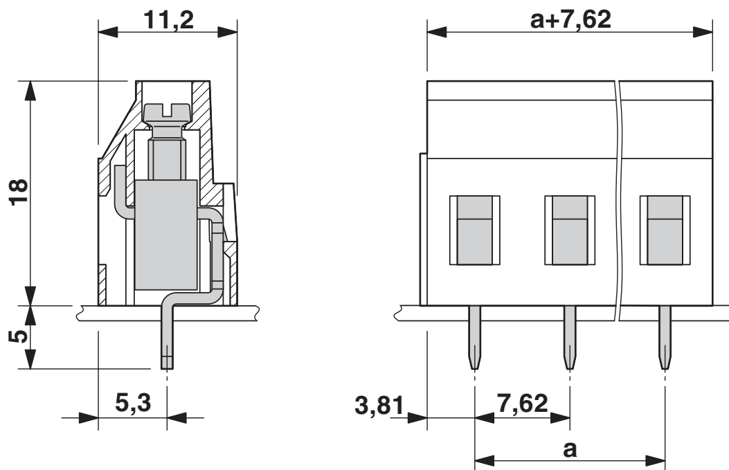
Måtskiss
