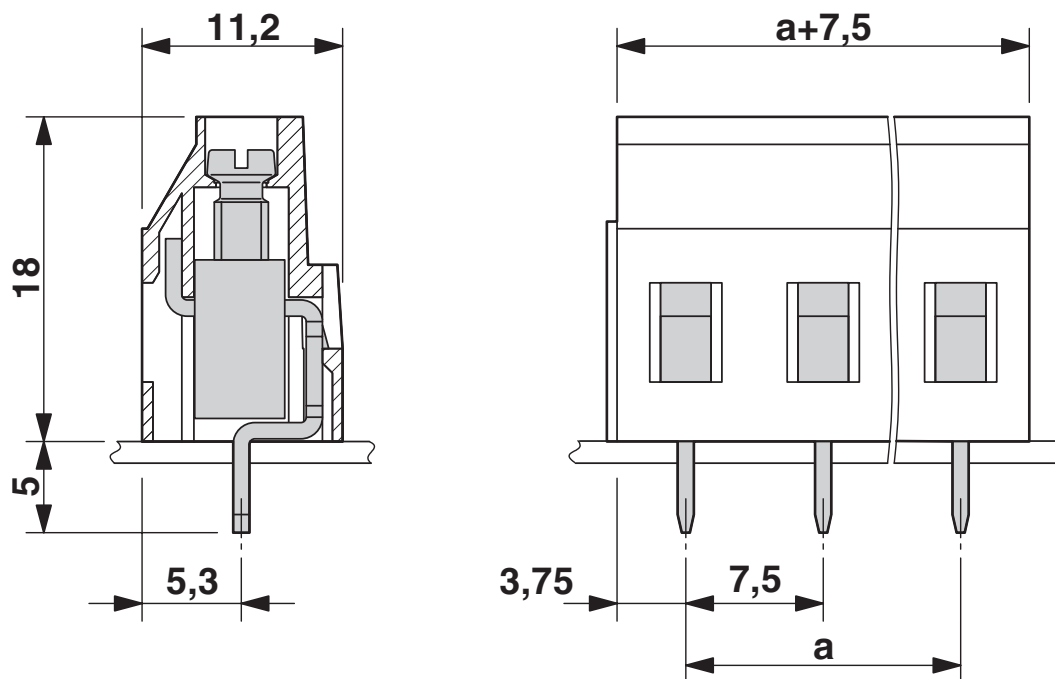
Måttskiss
