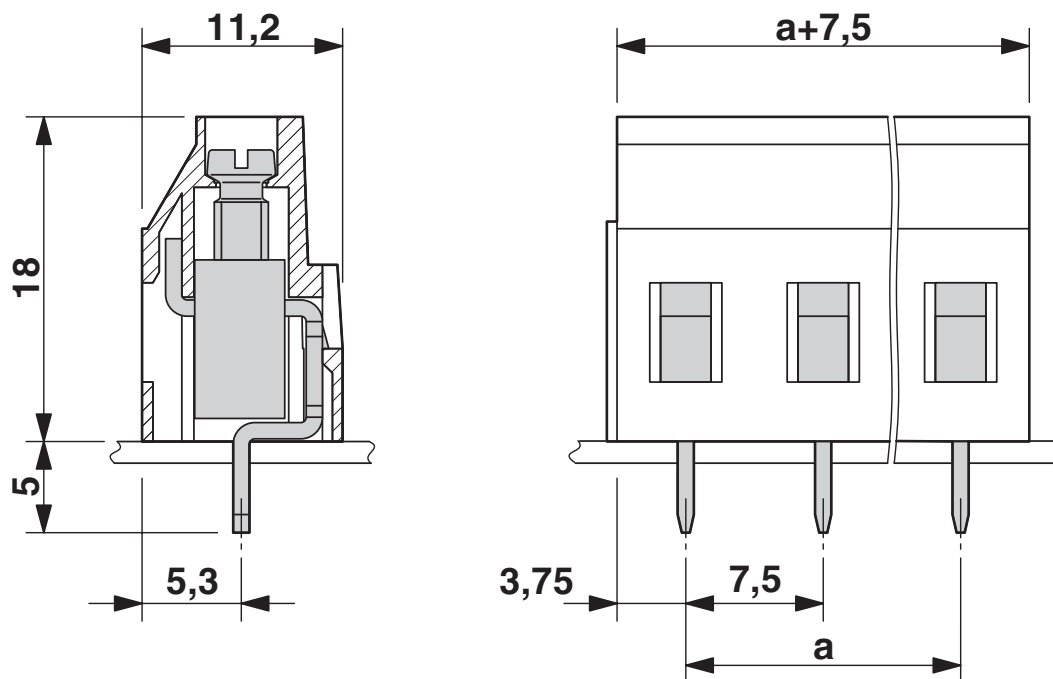
Måttskiss
