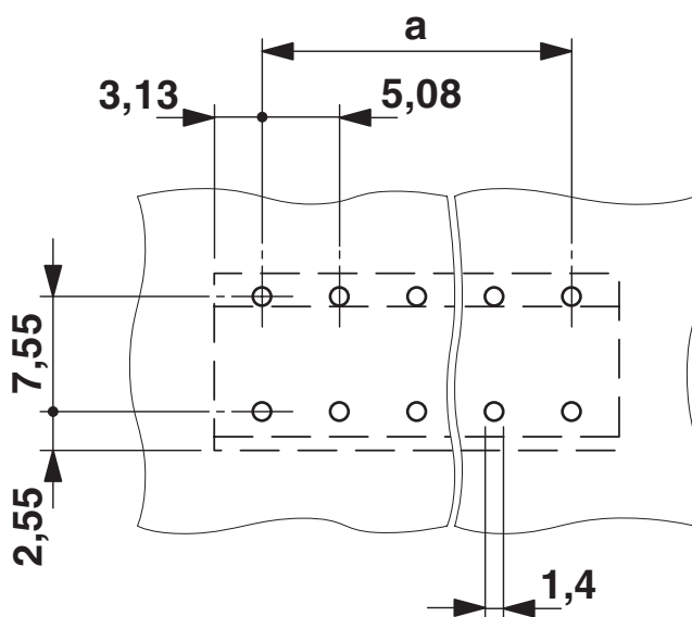
Borrplan/lödöns geometri
