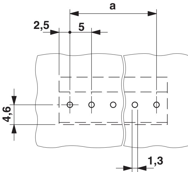
Borrplan/lödöns geometri
