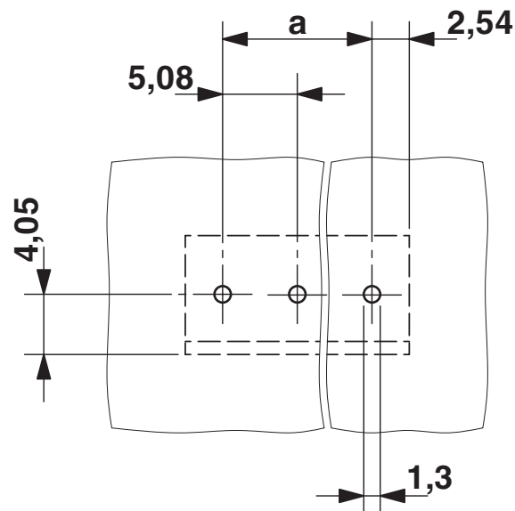
Borrplan/lödöns geometri
