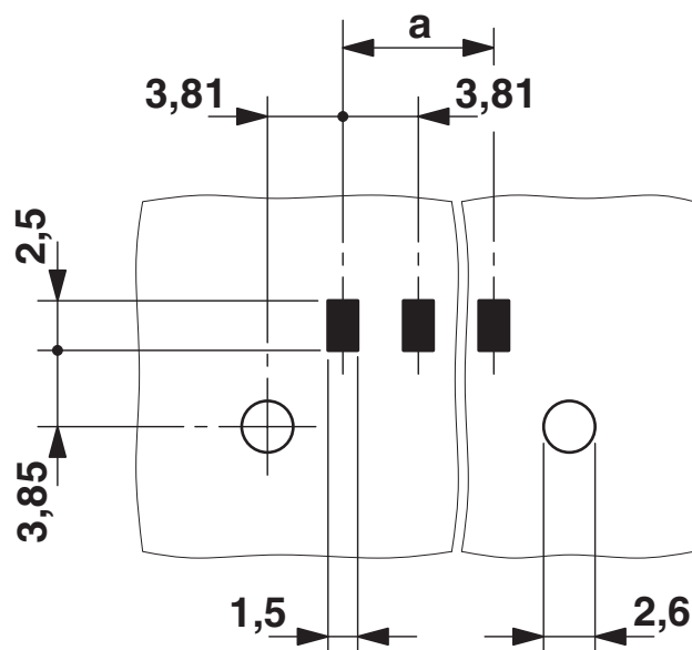
Borrplan/lödöns geometri
