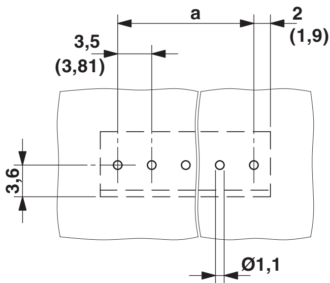
Borrplan/lödöns geometri
