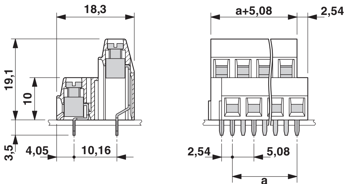
Måttskiss
