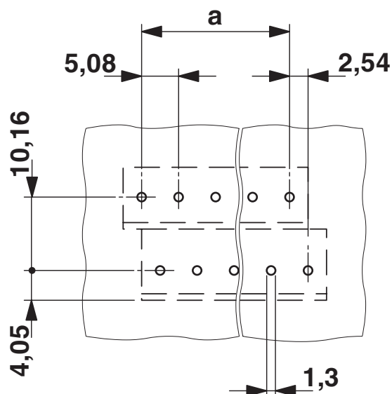
Borrplan/lödöns geometri
