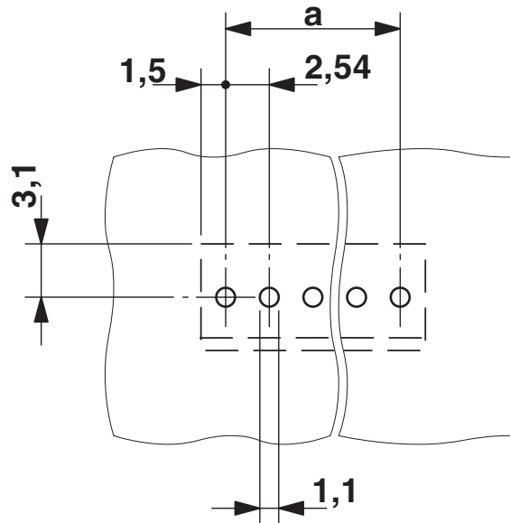
Borrplan/lödöns geometri
