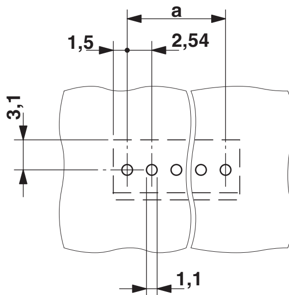
Borrplan/lödöns geometri
