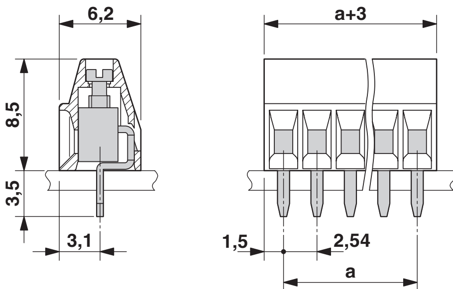
Måttskiss
