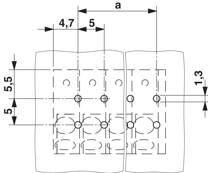
Borrplan/lödöns geometri
