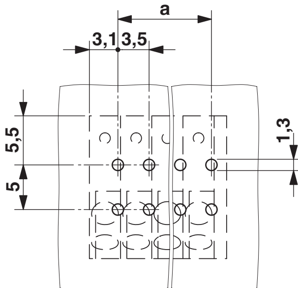
Borrplan/lödöns geometri
