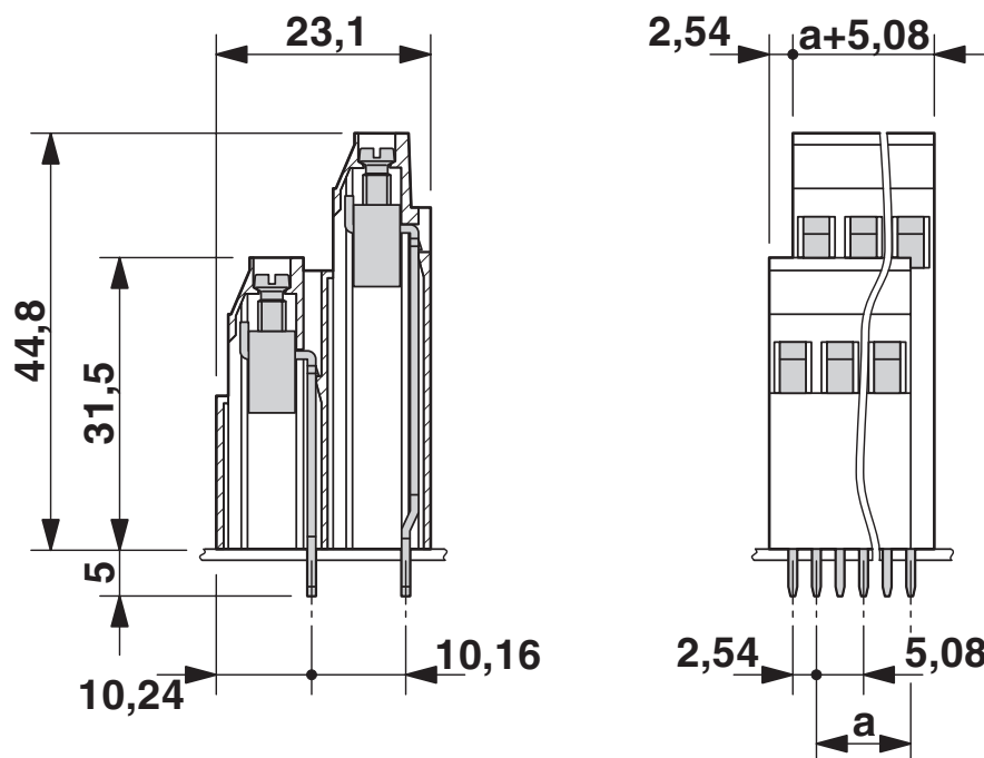
Måttskiss
