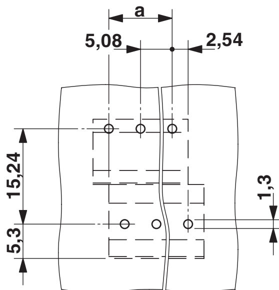
Borrplan/lödöns geometri
