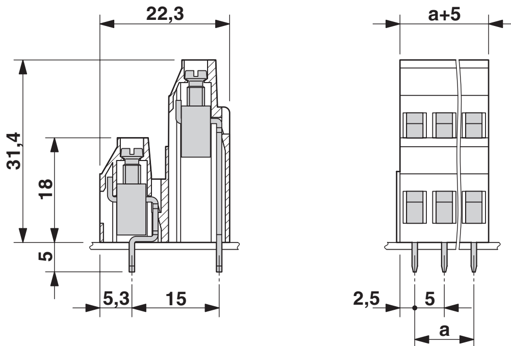
Måttskiss
