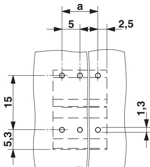
Borrplan/lödöns geometri
