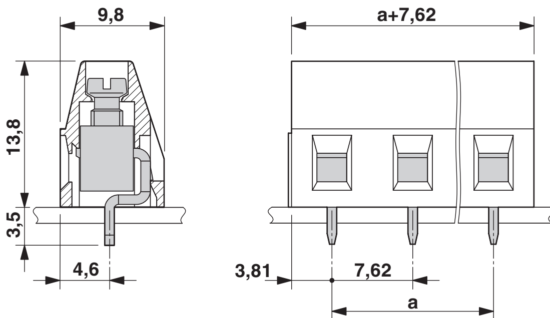
Måttskiss
