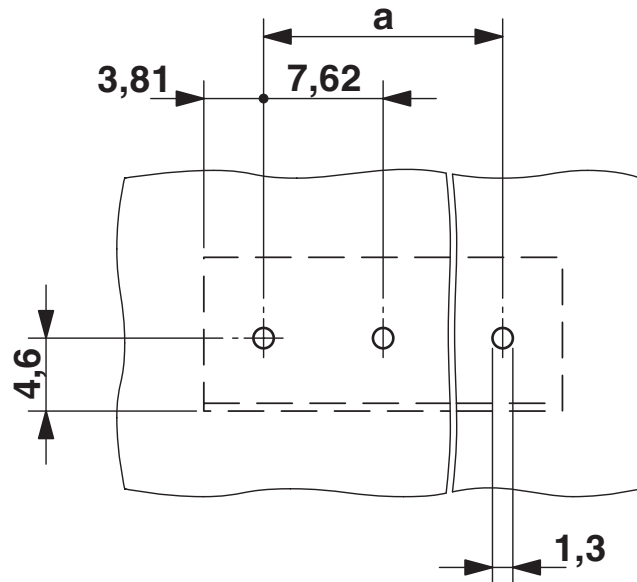
Borrplan/lödöns geometri
