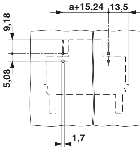
Borrplan/lödöns geometri
