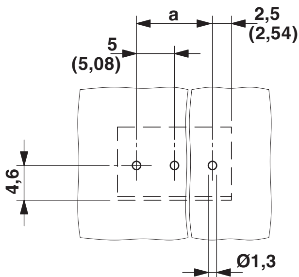
Borrplan/lödöns geometri
