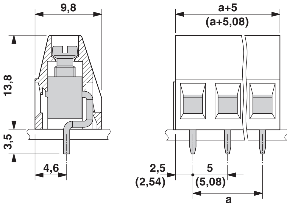
Måttskiss
