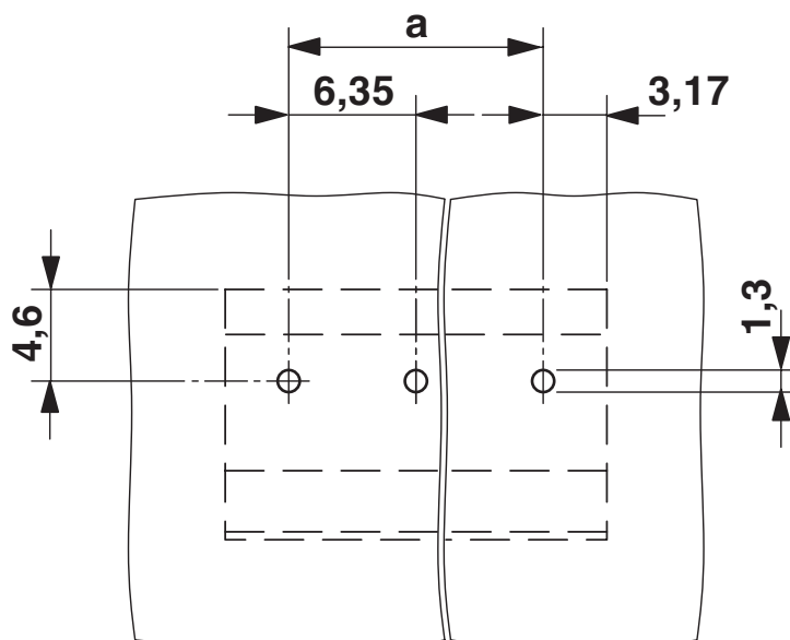
Borrplan/lödöns geometri
