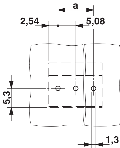
Borrplan/lödöns geometri
