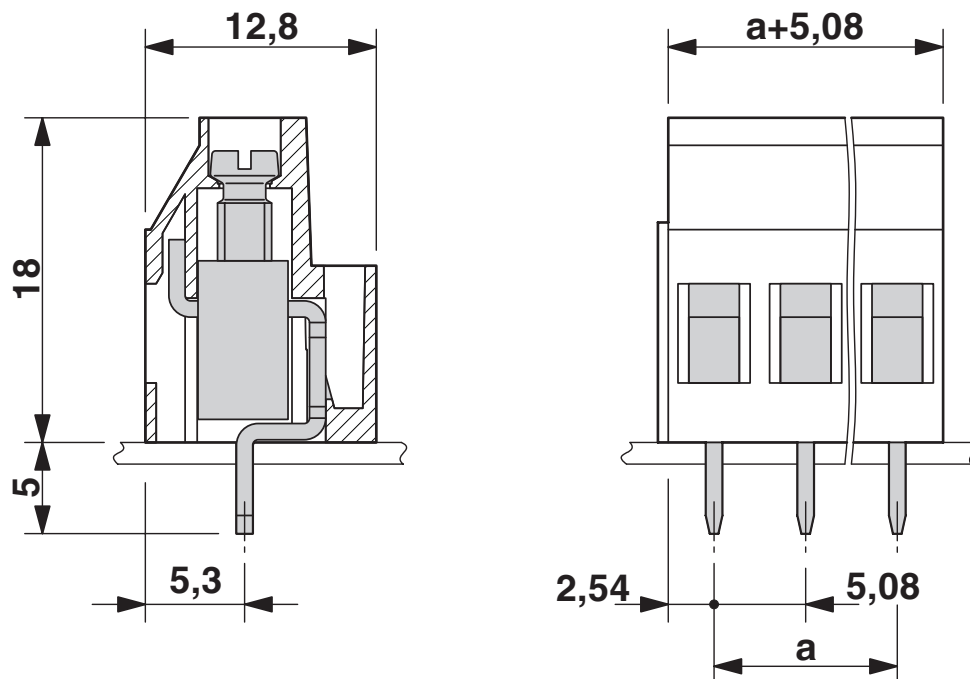
Måttskiss
