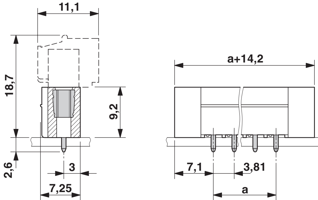
Måttskiss
