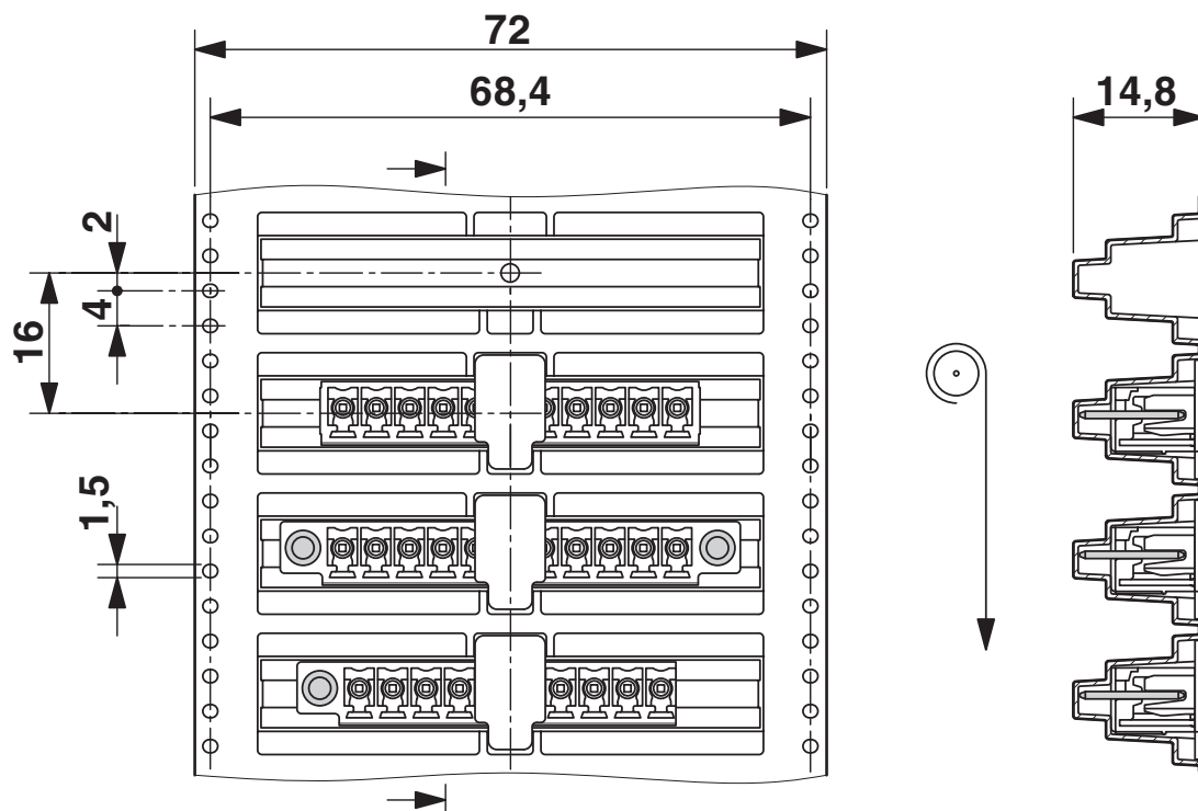
Måttskiss
