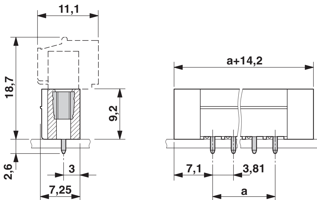
Måttskiss
