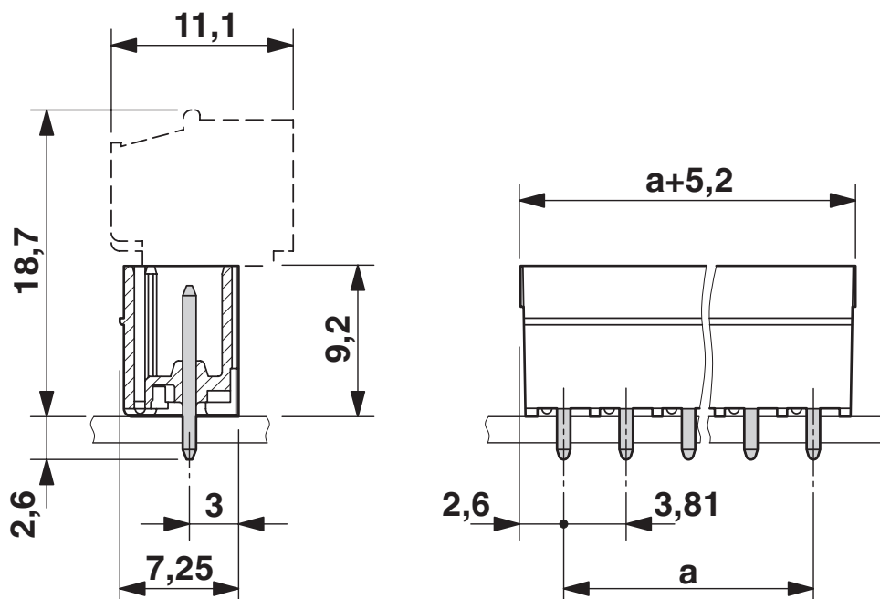
Måttskiss
