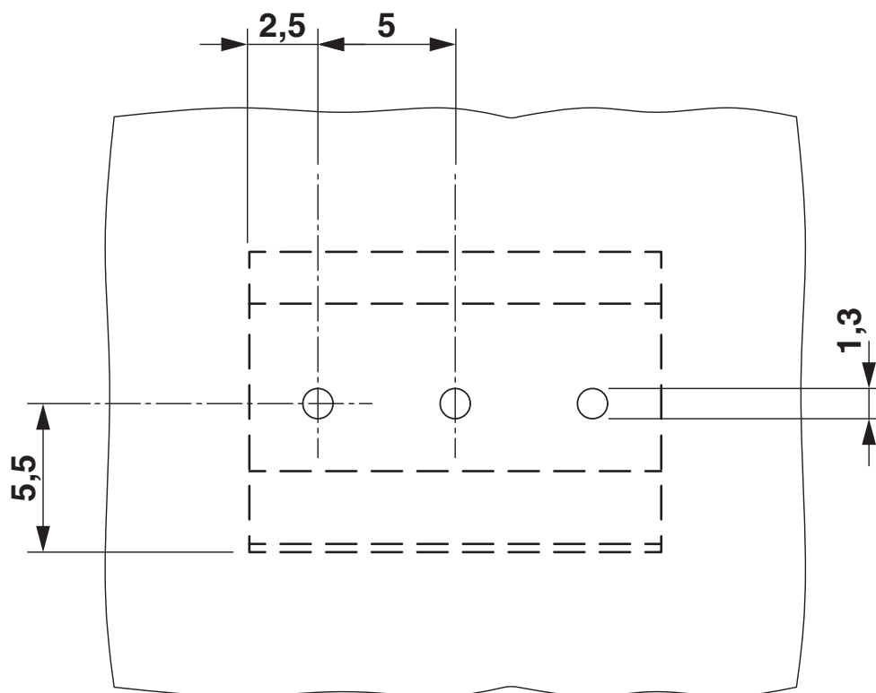
Borrplan/lödöns geometri
