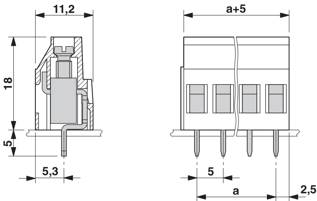
Måttskiss
