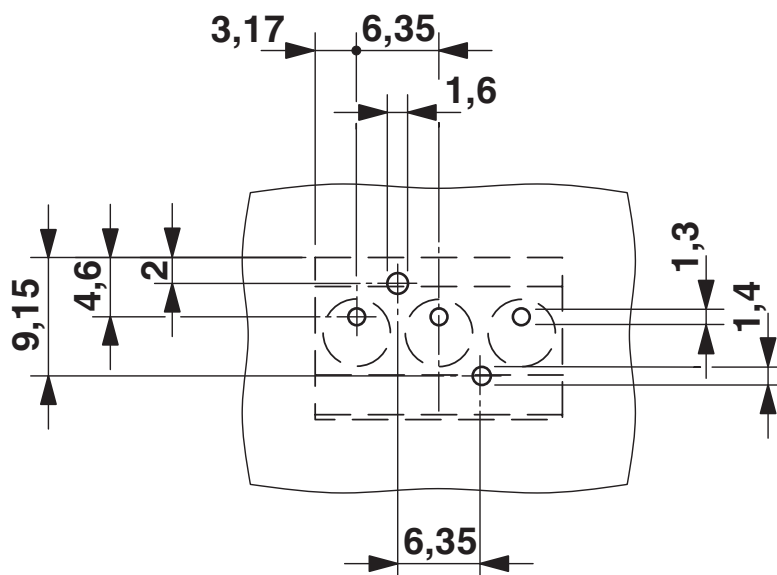
Borrplan/lödöns geometri
