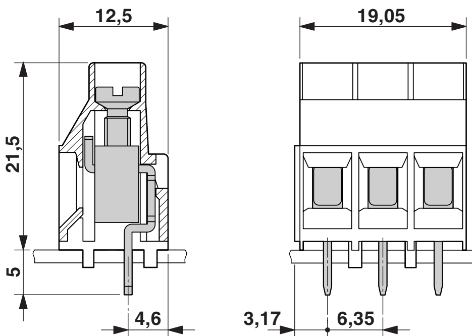
Måttskiss
