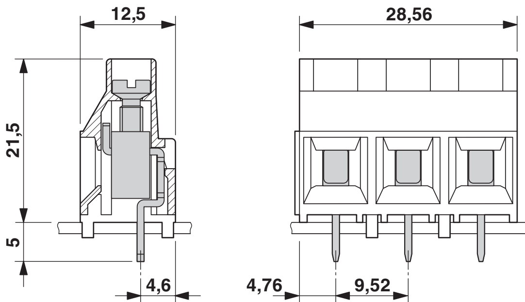
Måttskiss
