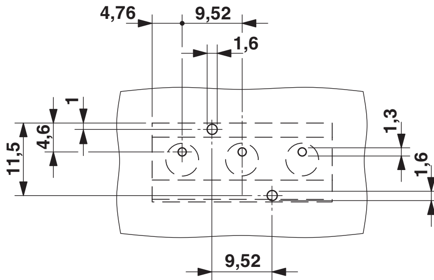
Borrplan/lödöns geometri
