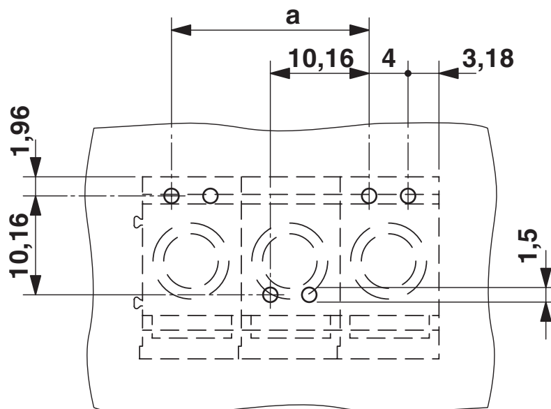
Borrplan/lödöns geometri
