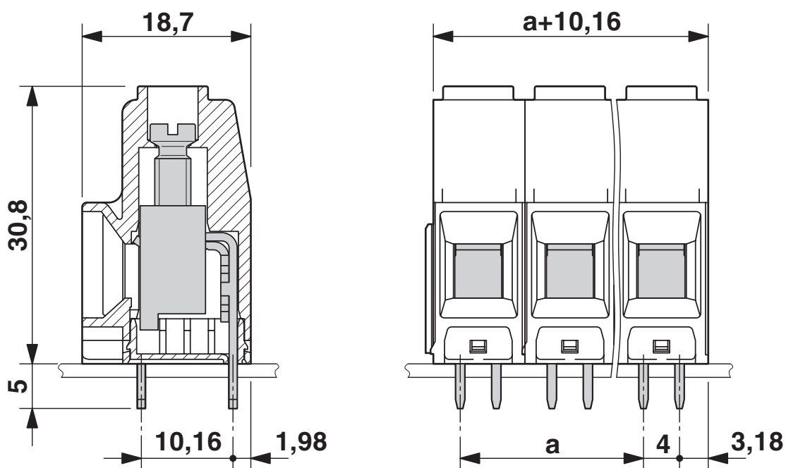
Måttskiss
