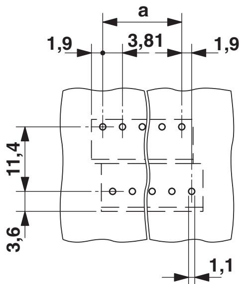
Borrplan/lödöns geometri
