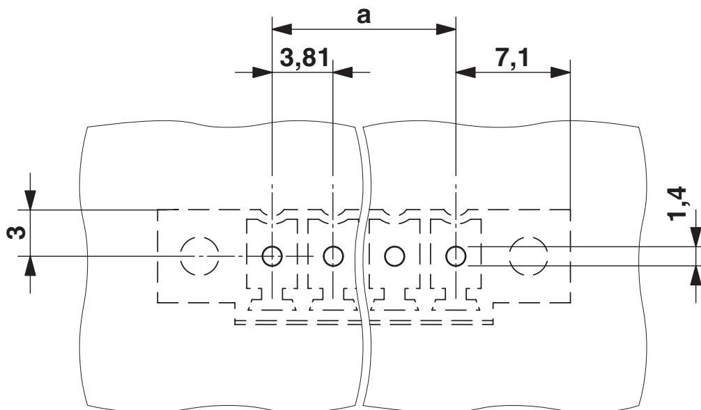
Borrplan/lödöns geometri
