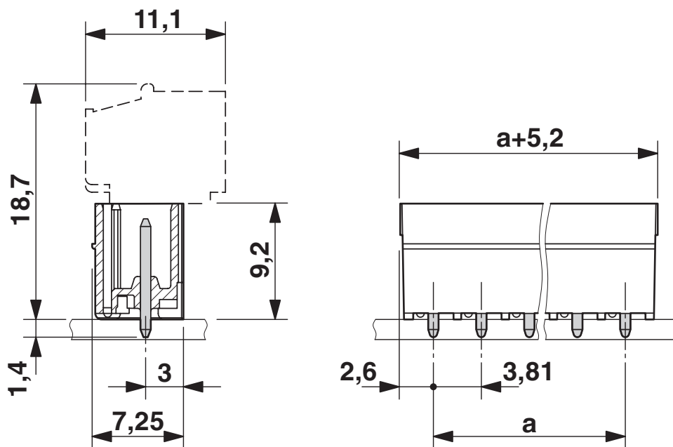
Måttskiss
