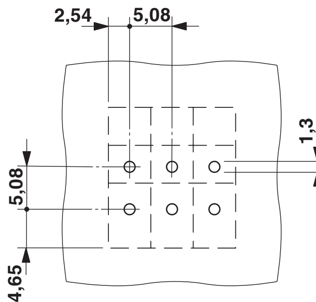
Borrplan/lödöns geometri
