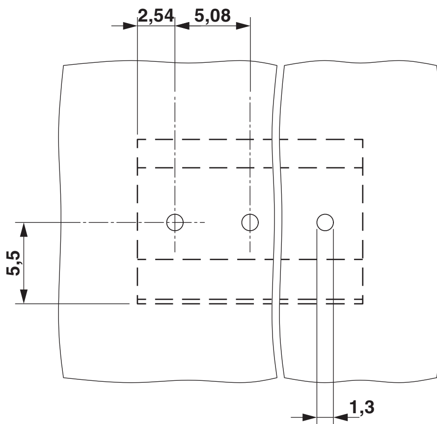
Borrplan/lödöns geometri
