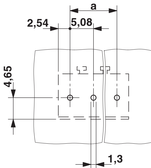
Borrplan/lödöns geometri
