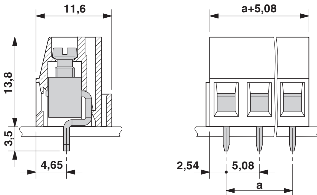
Måttskiss
